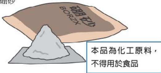
II. 硼砂
